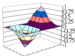
圖 1 邊界條件為 C-C-C-C 之第二模態
